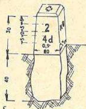
Obr. III/8. Doplňovací hraniční znak
