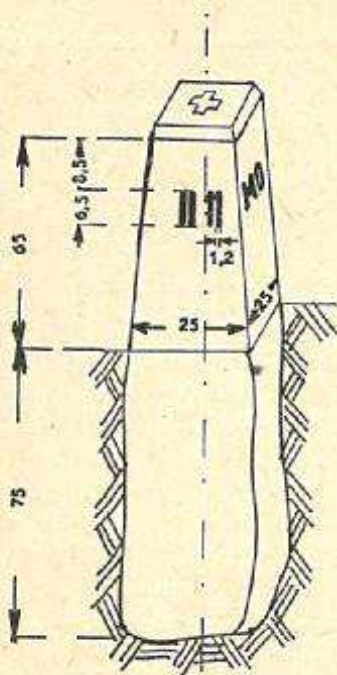
Obr. III/7. Hlavní hraniční znak
