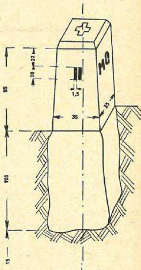
Obr. III/6. Základní hraniční znak
