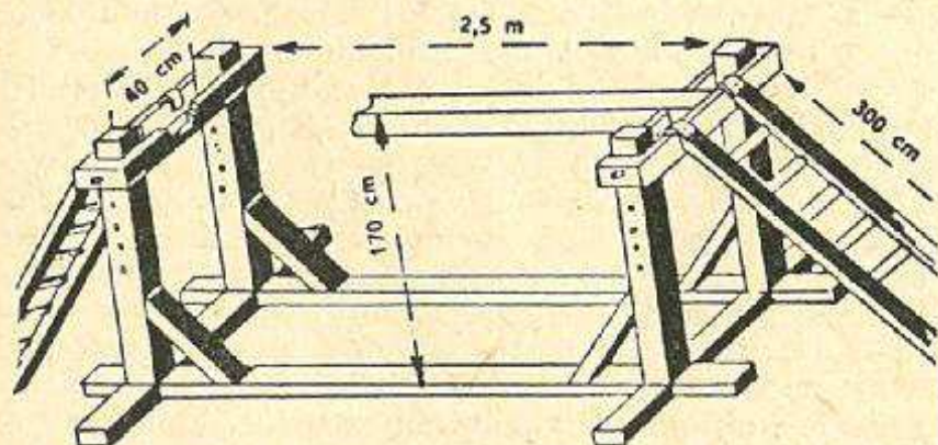
Obr. XI/2. Kladina se žebříky
